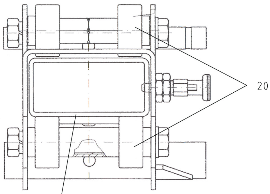
Fuehrungsschiene VA
