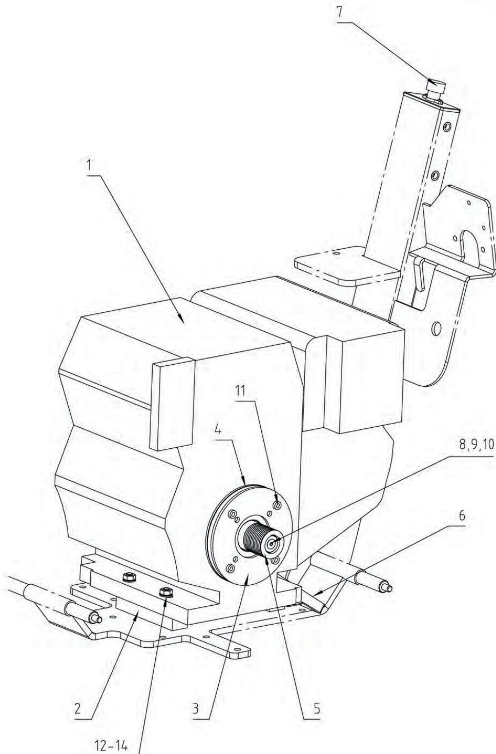
Aufbau - Benzinmotor Honda GX-390 Attachment gasoline engine Honda GX-390 CF-1010 B Pos. G
