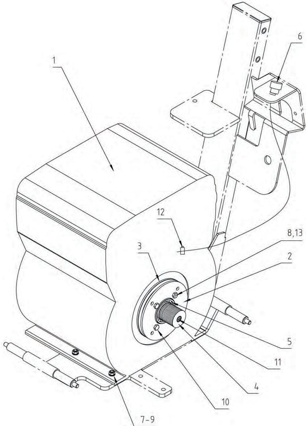
Aufbau Diesel-Motor Hatz 1B 40 Attachment Diesel engine Hatz 1B 40 CF-1010 D Pos.H
